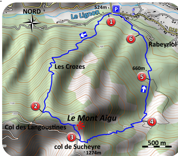
Carte IGN 2838 OT
